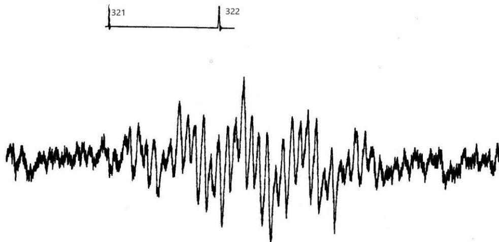
Рис. 2. Спектр ЭПР, полученный окислением липидного экстракта печени Squalus achantias диоксидом свинца в толуоле при 24°C, напряженность магнитного поля, мТл
